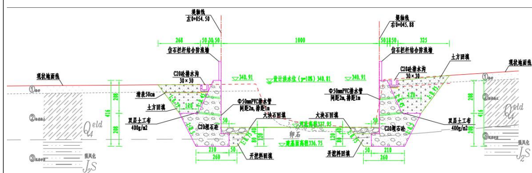
图 2-3 堤防结构典型横断面图(衡重式堤防)
