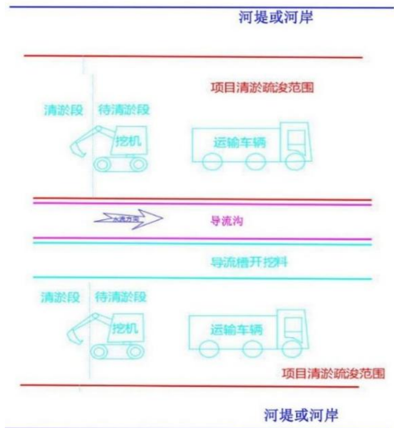
图 2.6-1 疏挖工程作业面示意图
