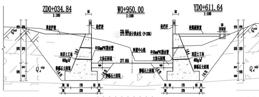
图 2-3 堤防结构典型横断面图（重力式堤防）
