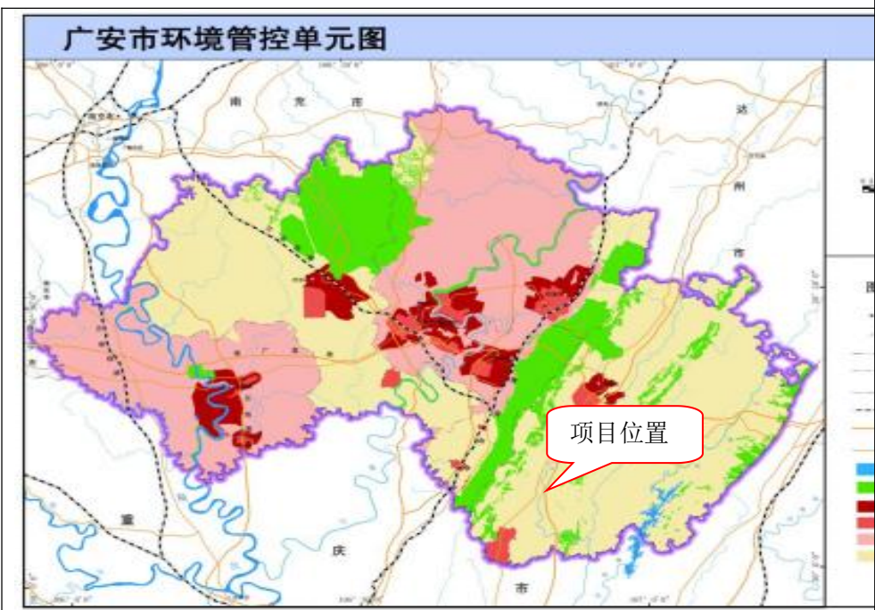
图 1-1 广安市环境管控单元划分图
