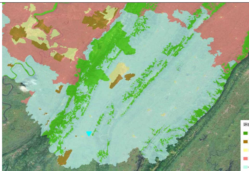
图 1-3 项目与环境综合管控单元的位置关系图（图中▼表示项目位置） 本项目与管控单元符合性分析详见下表 1.7-2。
